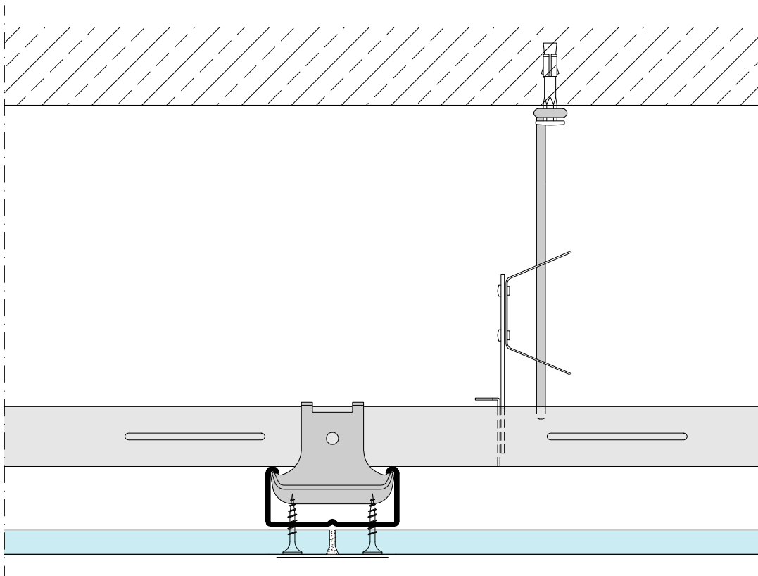
KNAUF D112.cz-C4 Styk řezaných hran - Nosný a montážní profil - rychlozávěs s drátem
