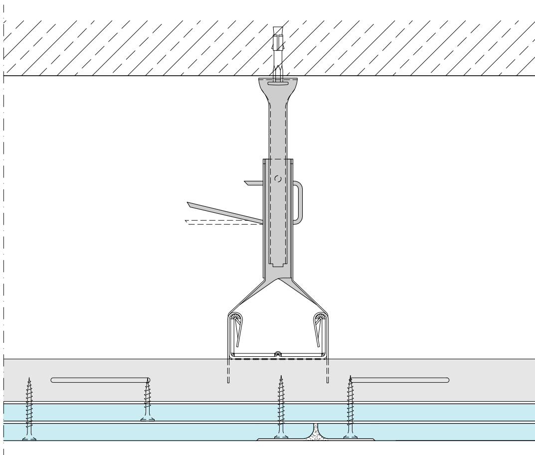
KNAUF D112.cz-B1 Styk podélných hran - Nosný a montážní profil - třmen noniusový CD
