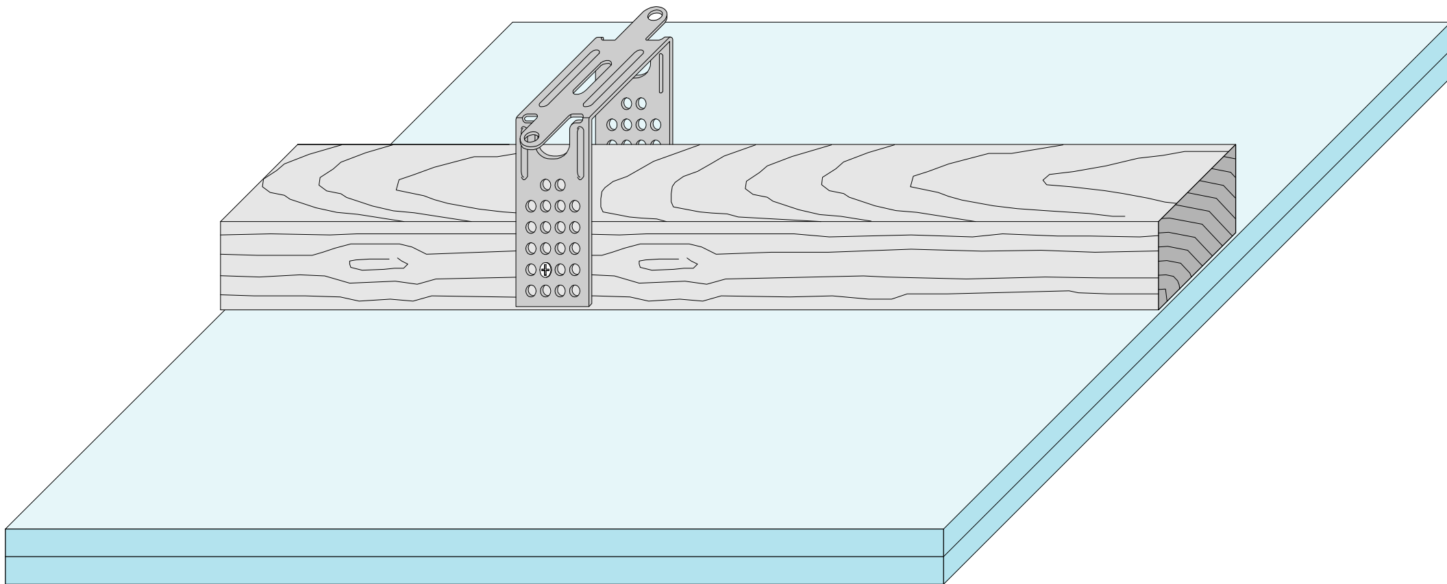
KNAUF D111.cz-P011 Perspektiva - montážní lať - přímý závěs
