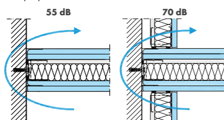
Napojení na obvodové konstrukce
