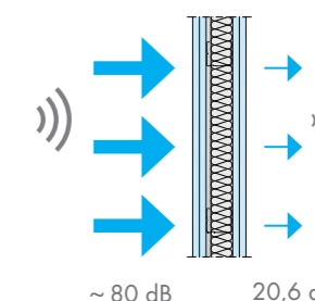
Dvojitě opláštěná sádrokartonová stěna Knauf
